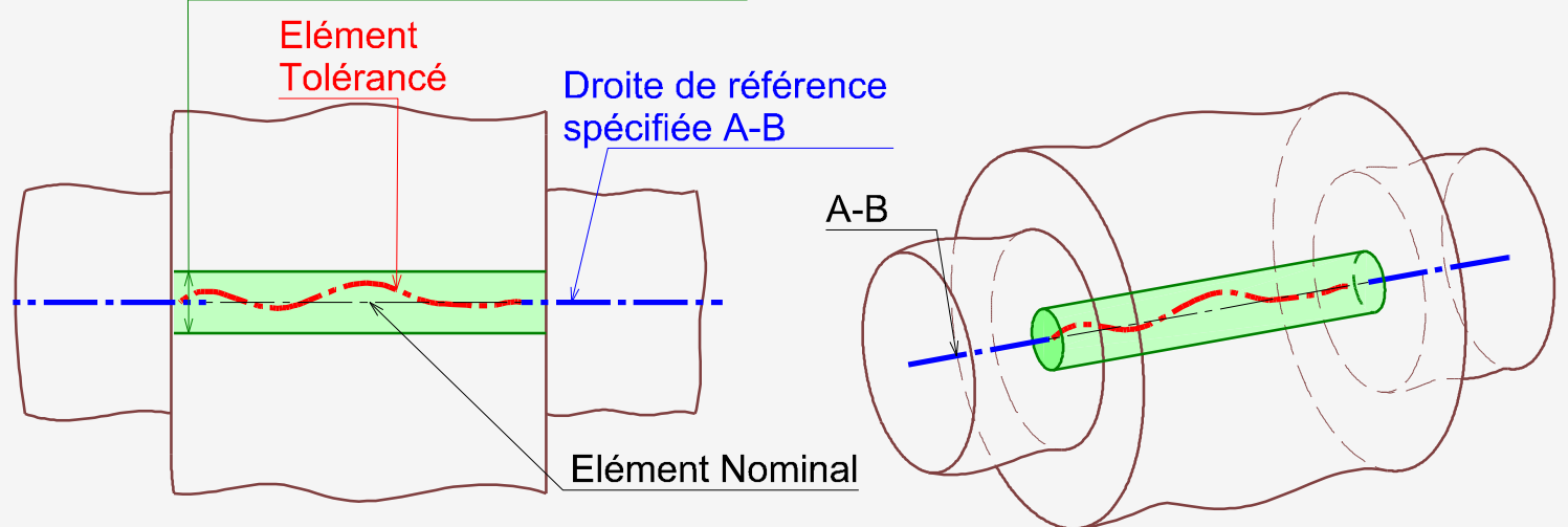
Zone de Tolérance de \phi 0.05 , centrée sur la droite de référence commune A-B
