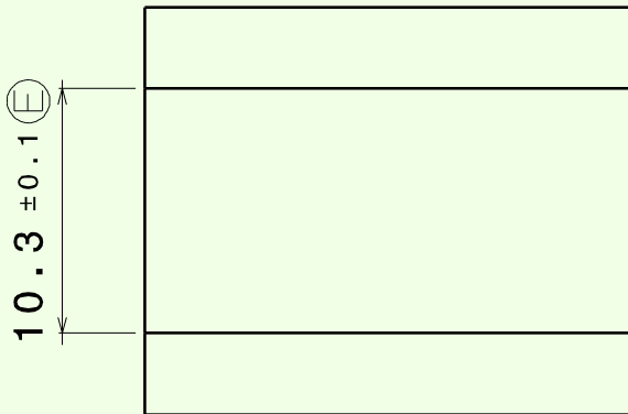
Exemple d'une rainure
