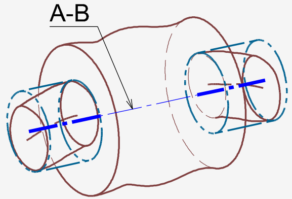
2 cylindres parfaitement coaxiaux circonscrits aux surfaces cylindriques réelles. Les éléments sont associés simultanément
