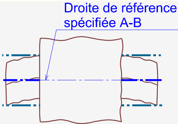
2 cylindres parfaitement coaxiaux circonscrits aux surfaces cylindriques réelles. Les éléments sont associés simultanément
