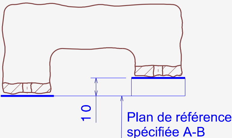
2 plans tangents extérieur matière parfaitement décalés de 10mm. Les éléments sont associés simultanément
