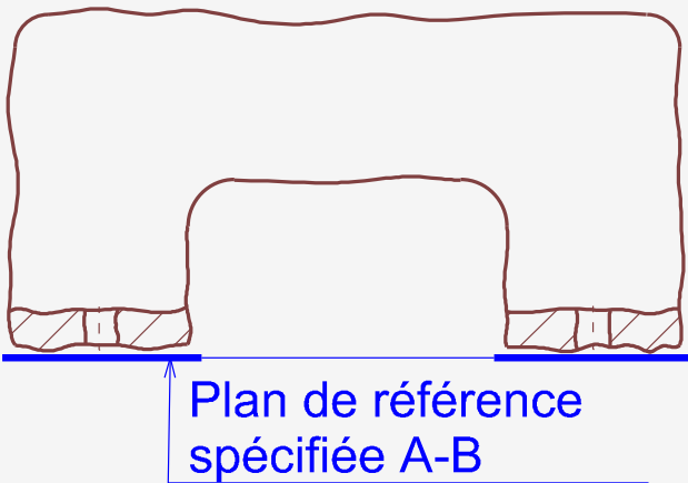
2 plans tangents extérieur matière parfaitement alignés. Les éléments sont associés simultanément
